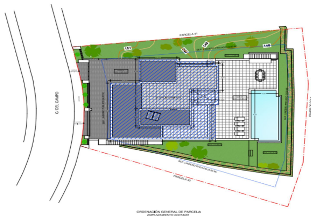
ORDENACIÓN GENERAL DE PARCELA: EMPLAZAMIENTO ACOTADO
